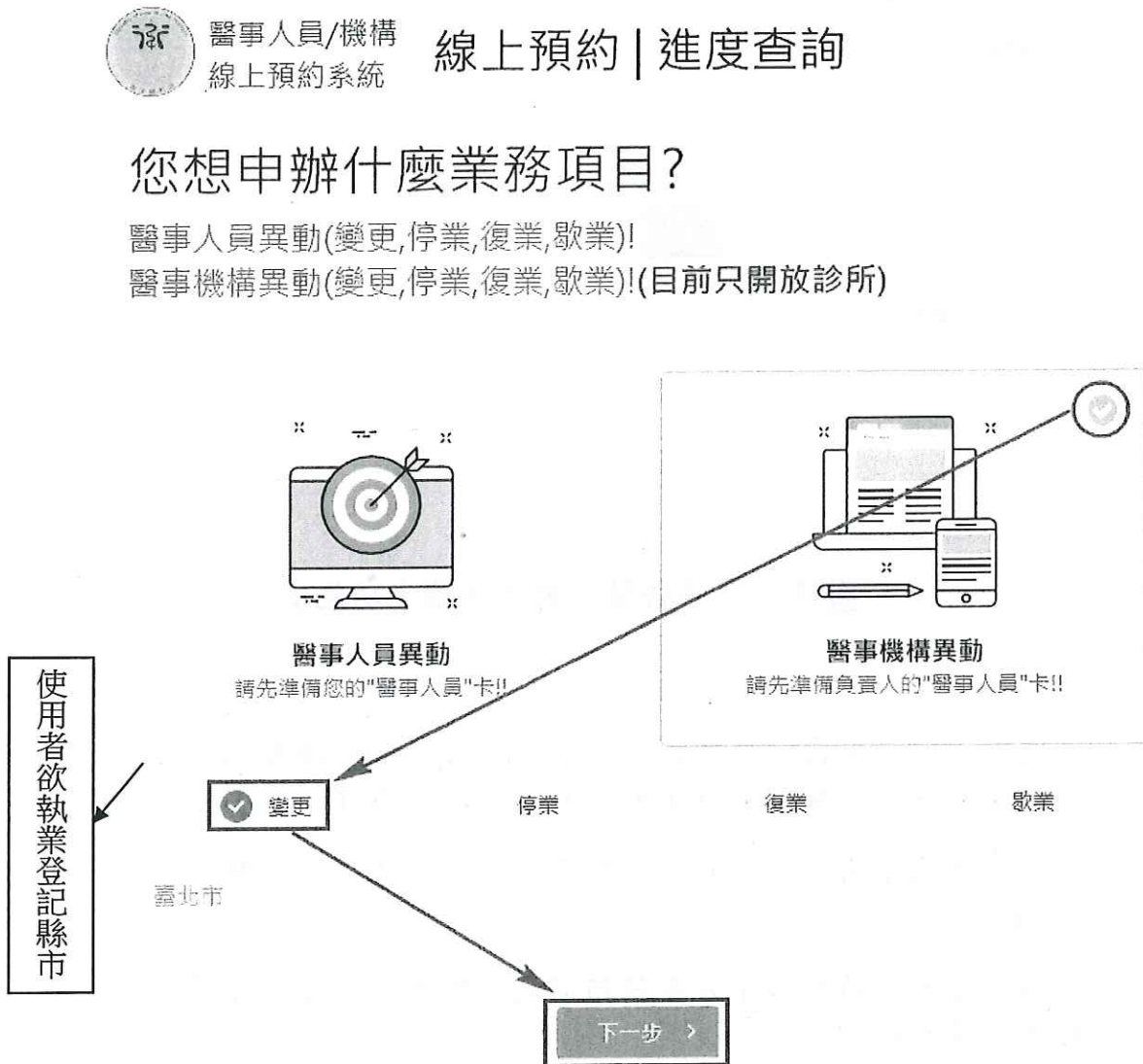
圖17 醫事機構異動變更操作畫面 1
